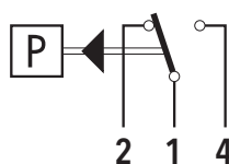
开关 21/26
